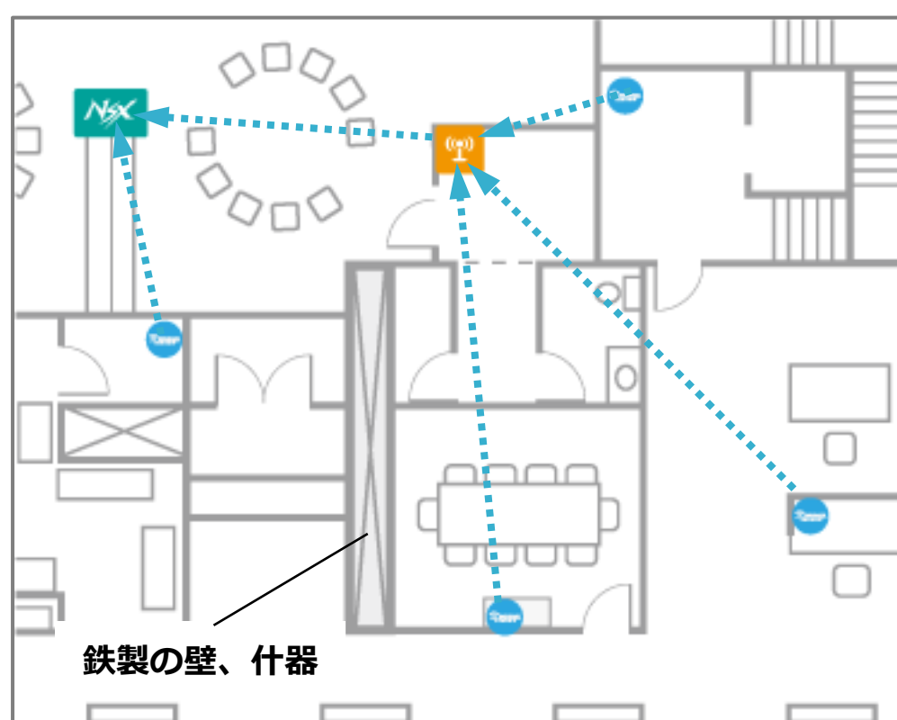
中継機を経由した場合の設置環境
