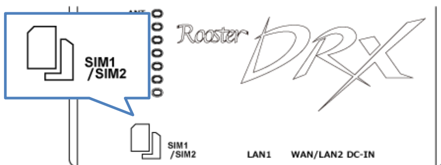
SIM1 の挿入口に入れる場合
