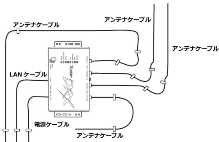
ケーブルの接続例（DRX5010,5510 の場合）
